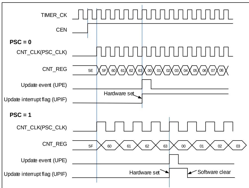
图 15-37. 向上计数时序图, PSC=0/1
