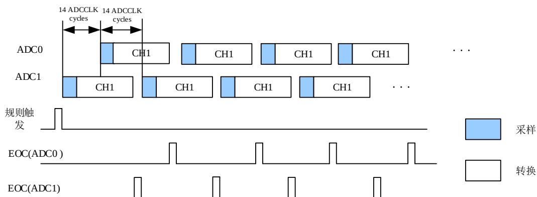
图 11-17. 一个采用连续转换模式通道上的慢速交叉模式
