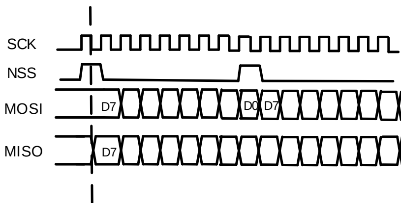
图 18-8. 主机 TI 模式在连续发送时的时序图
