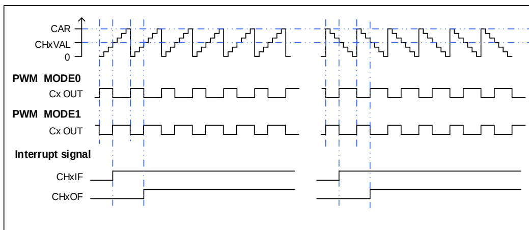
图 15-16. EAPWM 时序图
