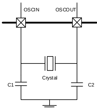
图5-3. HXTAL时钟源
