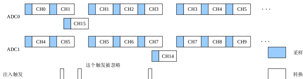
图 11-21. 在注入转换过程中触发出现
