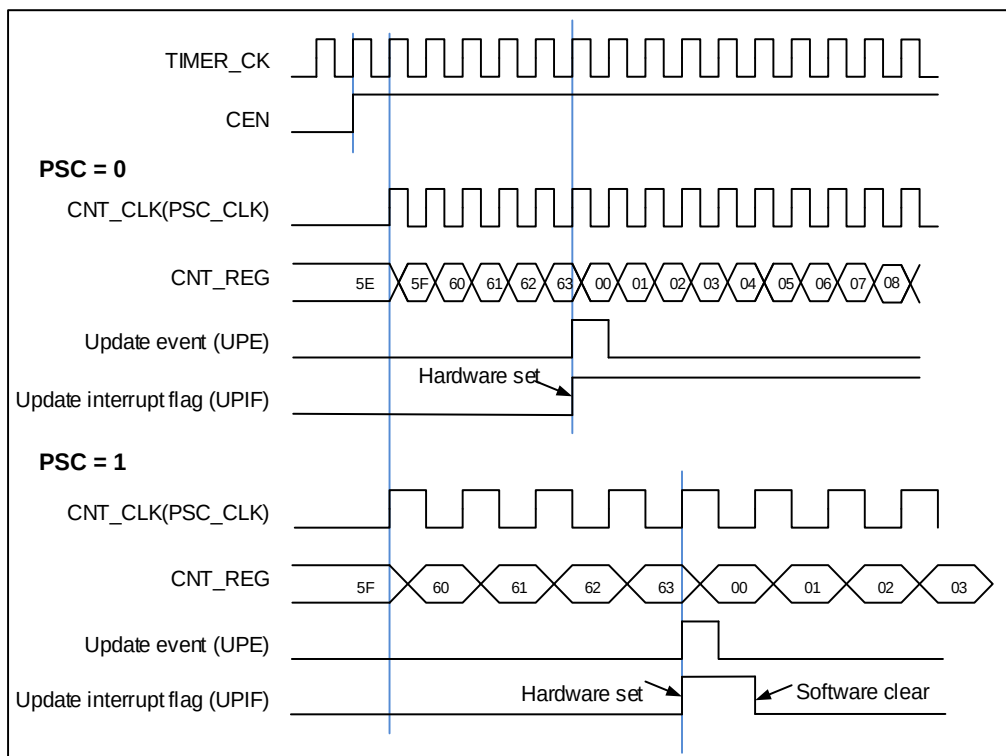
图 15-4. 向上计数时序图, PSC=0/1
