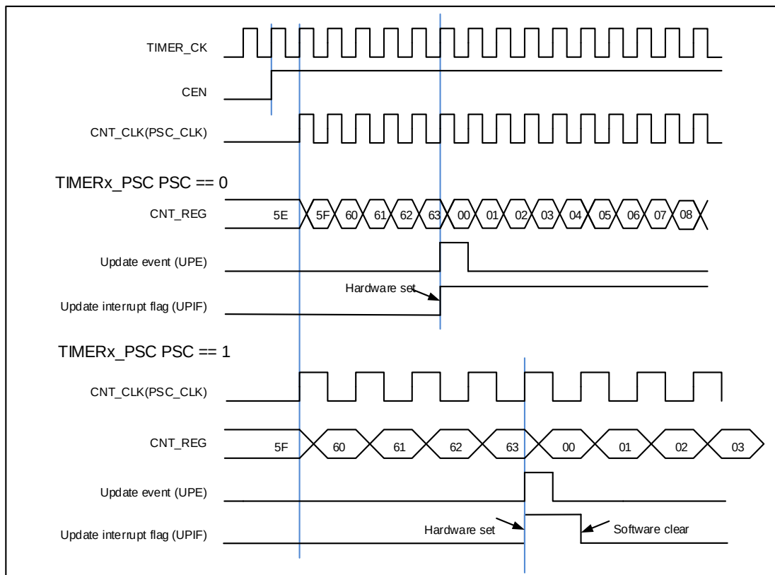
图 15-55. 向上计数时序图, PSC=0/1
