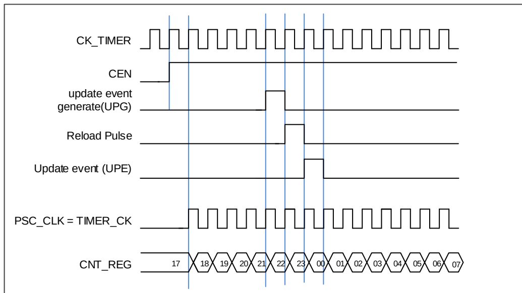
图 15-2. 内部时钟分频为 1 时，正常模式下的控制电路
