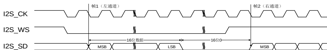
图 18-19. I2S 飞利浦标准时序图 (DTLEN=00, CHLEN=1, CKPL=1)
