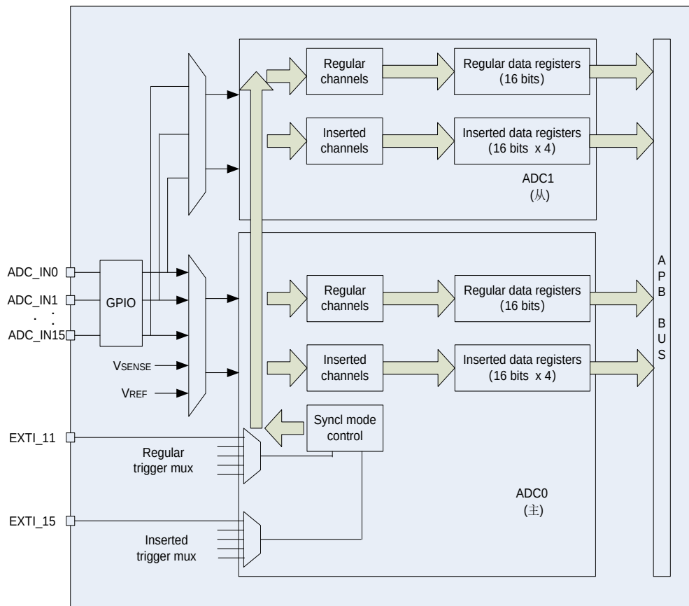
图 11-13. ADC 同步框图
