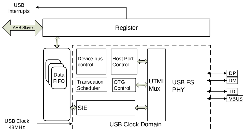
图 21-1. USBFS 结构框图
