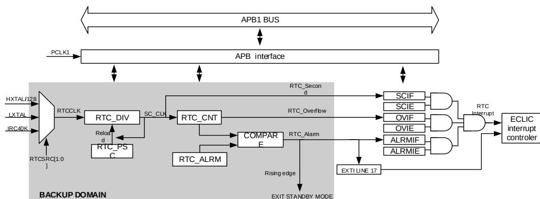
图 14-1. RTC 框图
