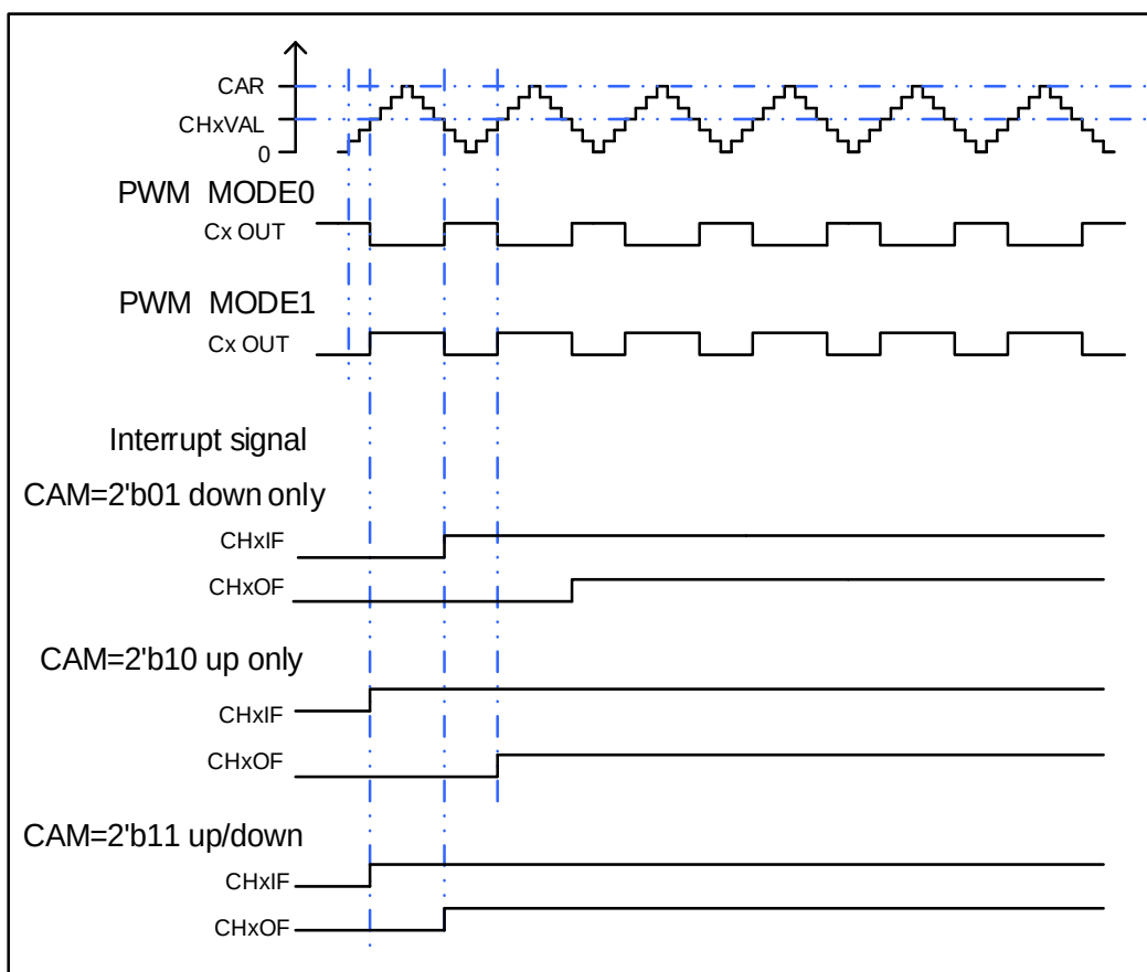
图 15-17. CAPWM 时序图
