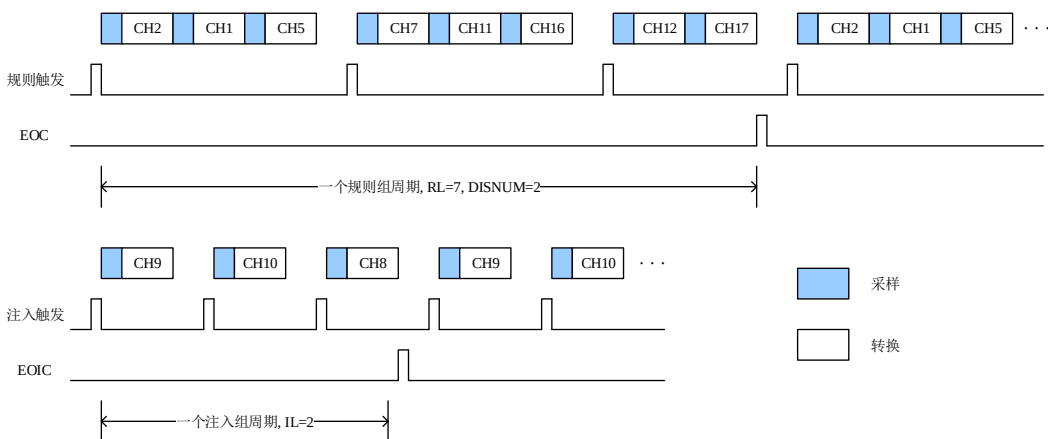
图 11-6. 中断转换模式
