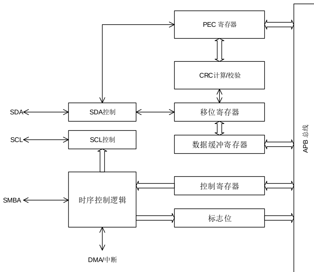
图 17-1. I2C 模块框图
