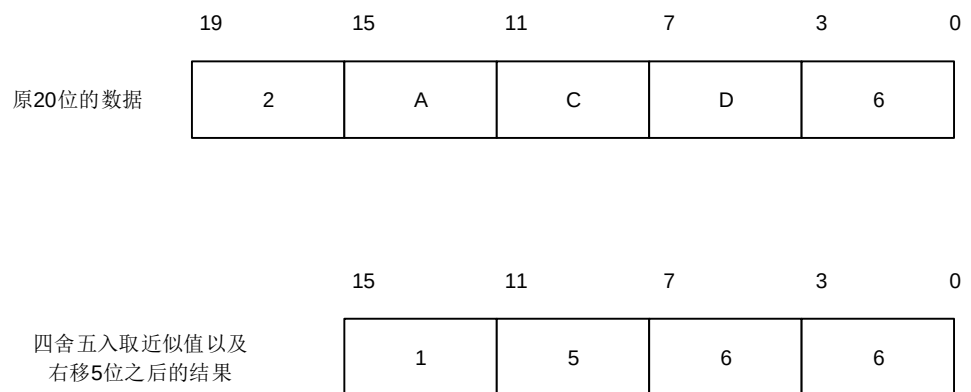
图 11-12. 右移 5 位和取整的数例
