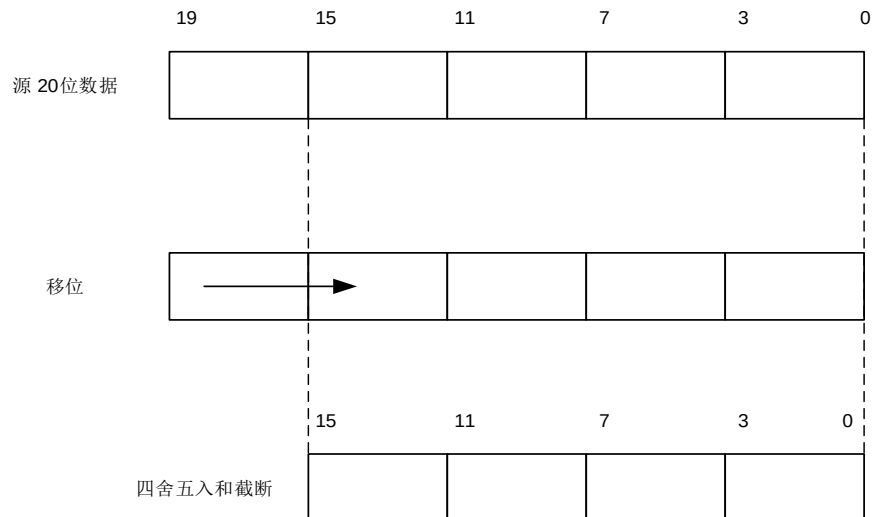
图 11-11. 20 位到 16 位的结果截断
