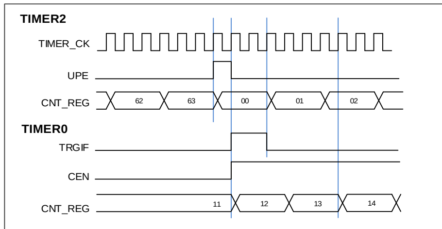
图 15-30. 用定时器 2 的更新事件来触发定时器 0
