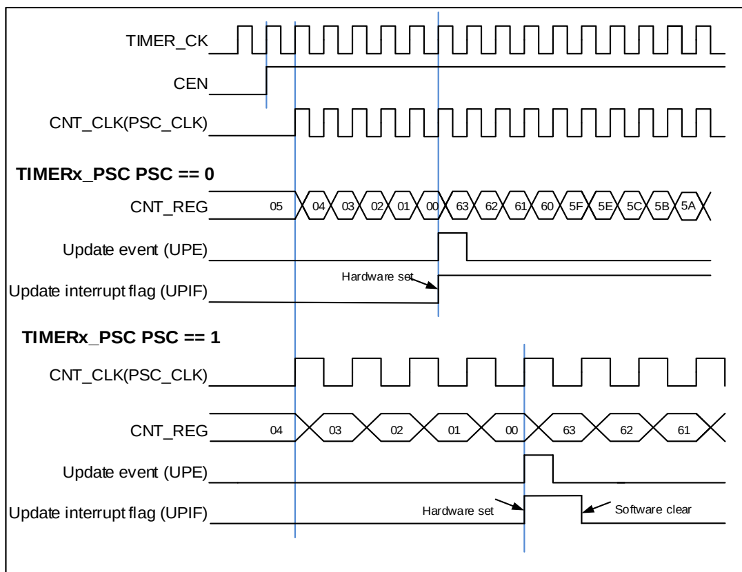
图 15-6. 向下计数时序图, PSC=0/1
