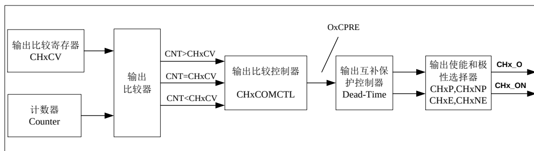
图 15-13. 输出比较逻辑（带有互补输出的通道， x=0,1,2 ）
