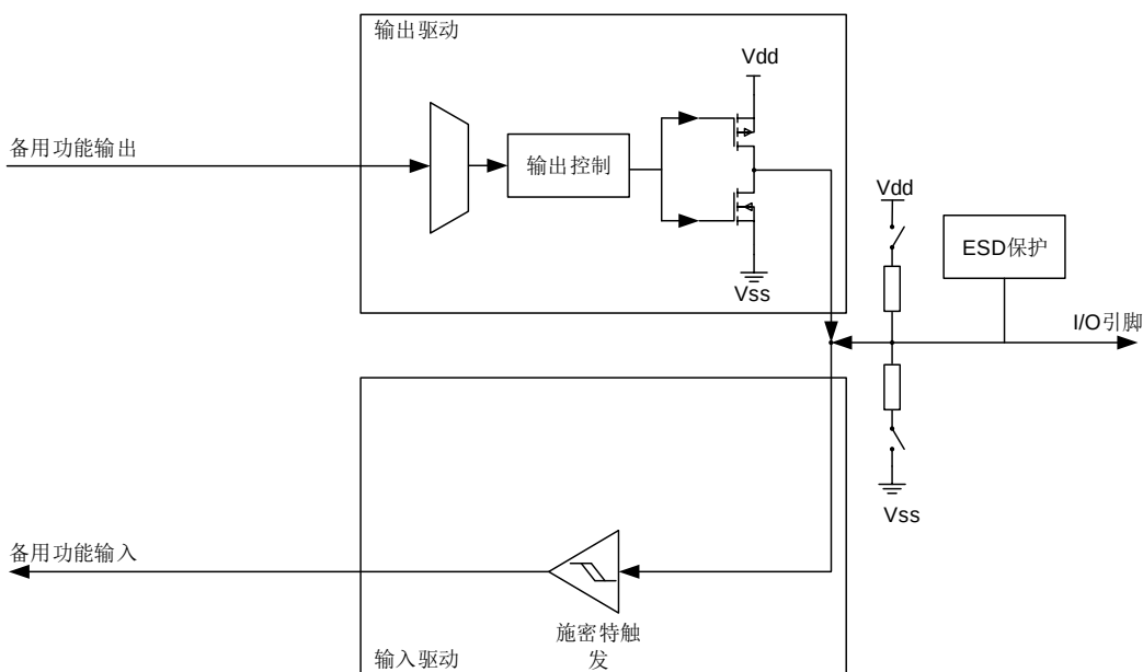
图 7-5. 备用功能配置
