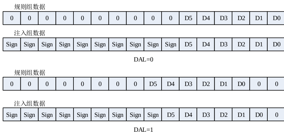
图 11-10. 6 位数据对齐
