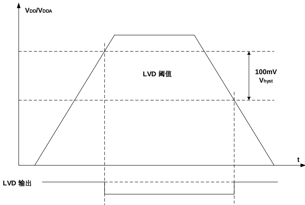
图 3-3. LVD 阈值波形图
