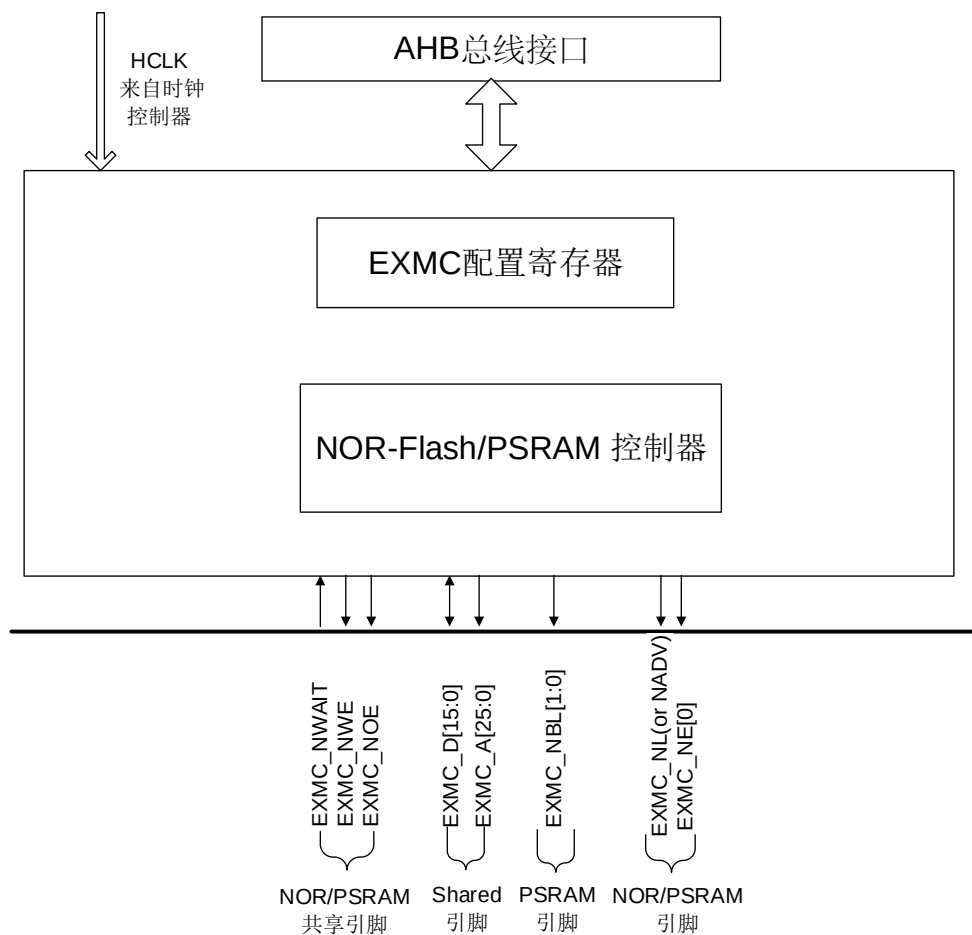
图 19-1. 系统架构
