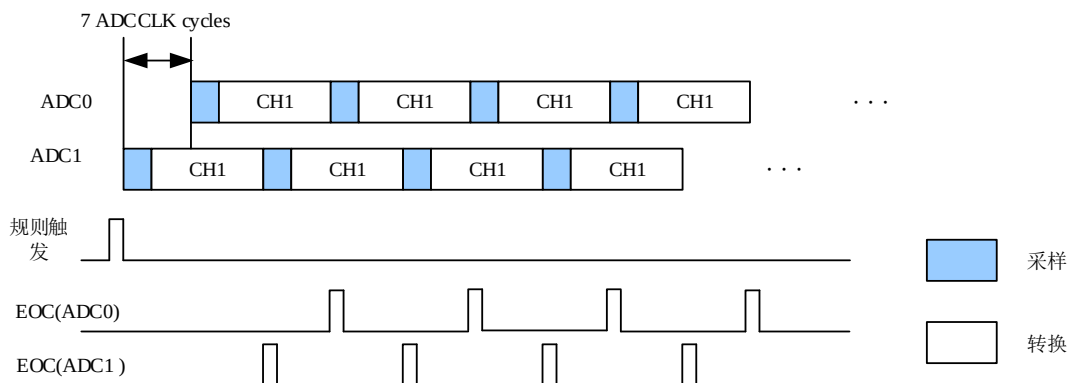
图 11-16. 一个采用连续转换模式通道上的快速交叉模式
