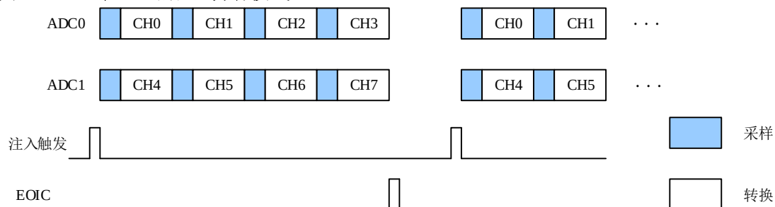
图 11-15. 4 个通道的注入并行模式
