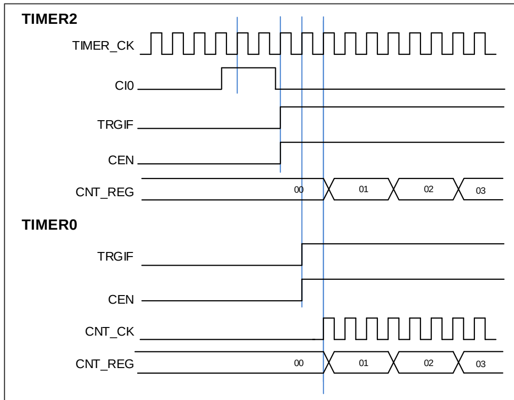
图 15-33. 用定时器 2 的 CI0 信号来触发定时器 0 和定时器 2
