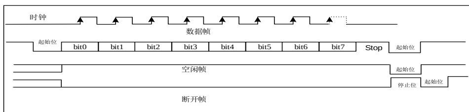
图 16-2. USART 字符帧 (8 数据位和 1 停止位)
