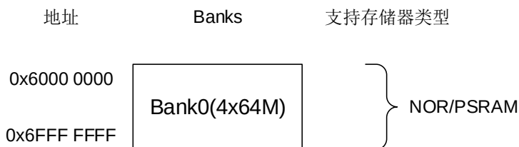
图 19-2. EXMC Bank 划分
