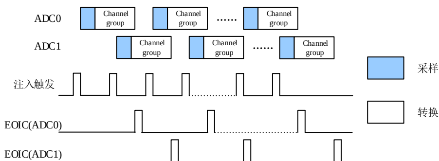
图 11-18. 交替触发: 注入通道组
