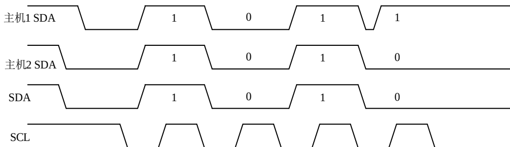
图 17-5. SDA 线仲裁
