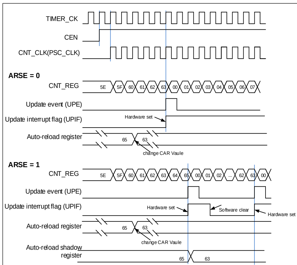
图 15-38. 向上计数时序图, 在运行时改变TIMERx_CAR寄存器的值
