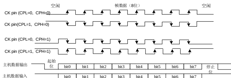
图 16-12. 8-bit 格式的 USART 同步通信波形(CLEN=1)
