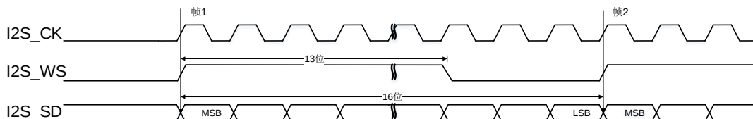
图 18-40. PCM 标准长帧同步模式时序图 (DTLEN=00, CHLEN=0, CKPL=0)
