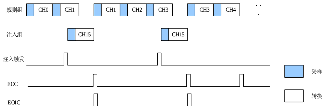
图 11-8. 触发注入
