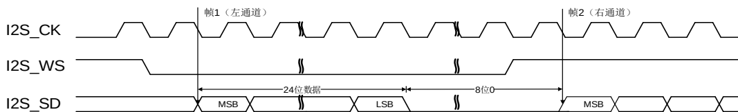
图 18-16. I2S 飞利浦标准时序图 (DTLEN=01, CHLEN=1, CKPL=0)
