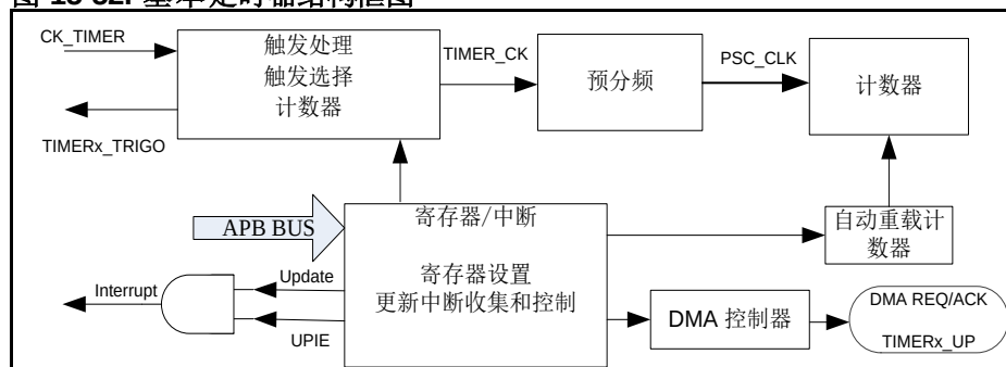
图 15-52. 基本定时器结构框图
