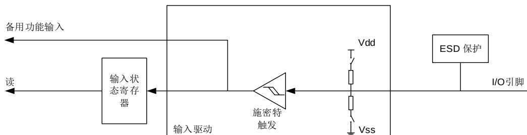
图 7-2. 输入配置
