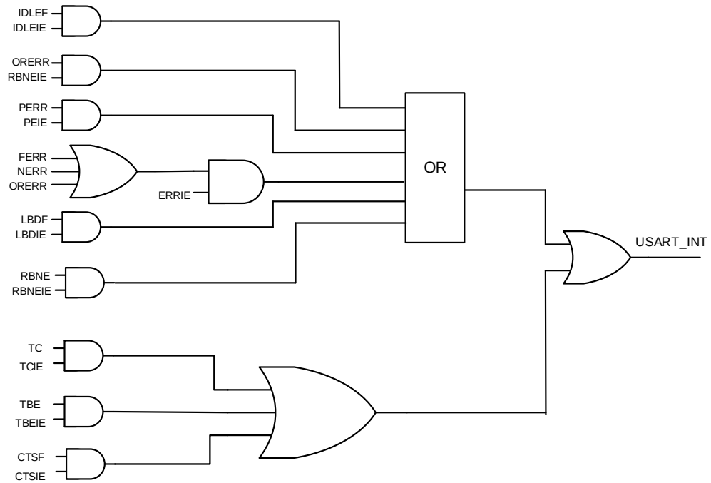
图 16-16. USART 中断映射框图
