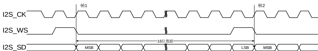
图 18-33. PCM 标准短帧同步模式时序图 (DTLEN=00, CHLEN=0, CKPL=1)
