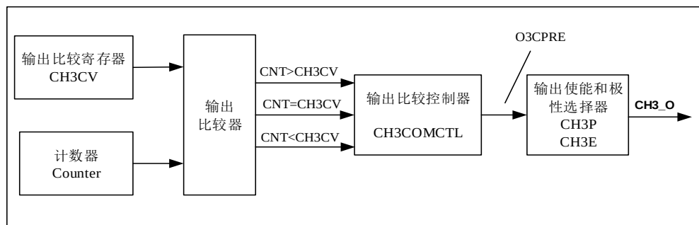
图 15-14. 输出比较逻辑
