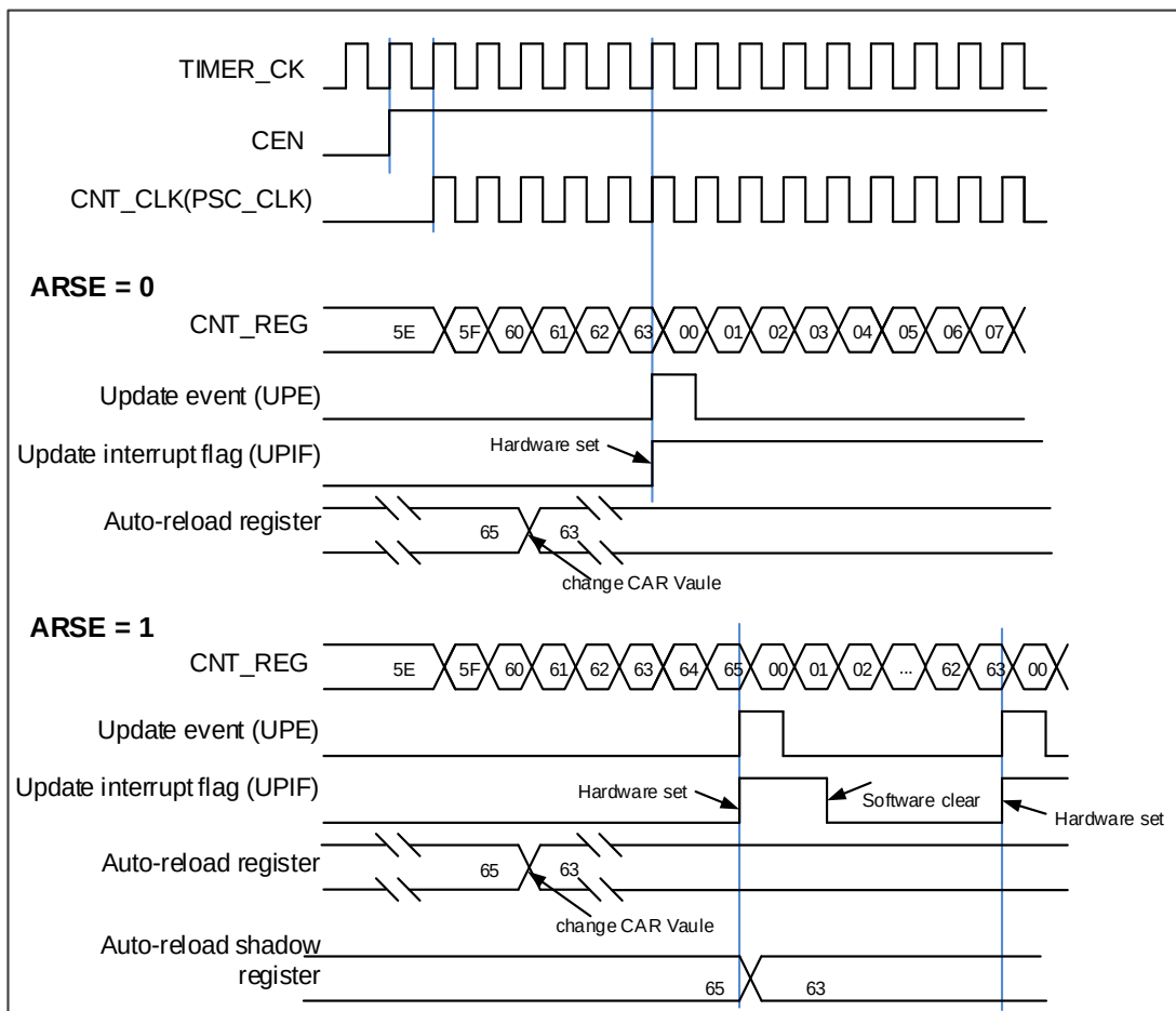
图 15-56. 向上计数时序图，在运行时改变 TIMERx_CAR 寄存器的值
