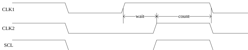
图 17-4. 时钟同步
