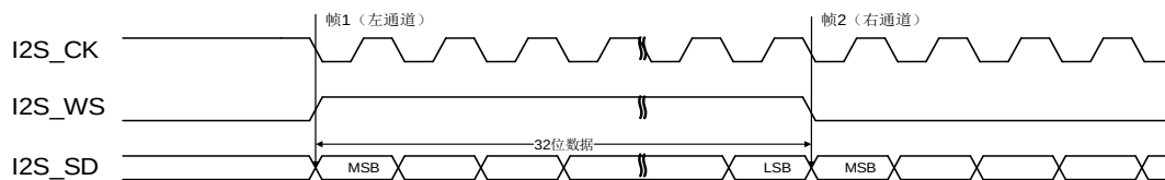
图 18-23. MSB 对齐标准时序图 (DTLEN=10, CHLEN=1, CKPL=1)
