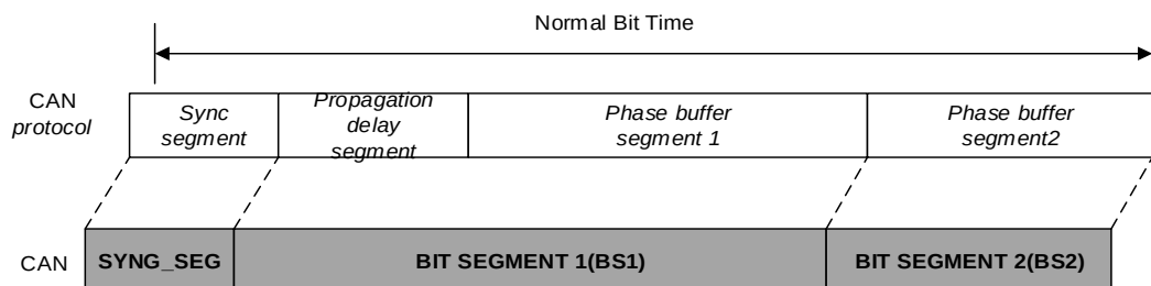
图 20-11. 位时序
