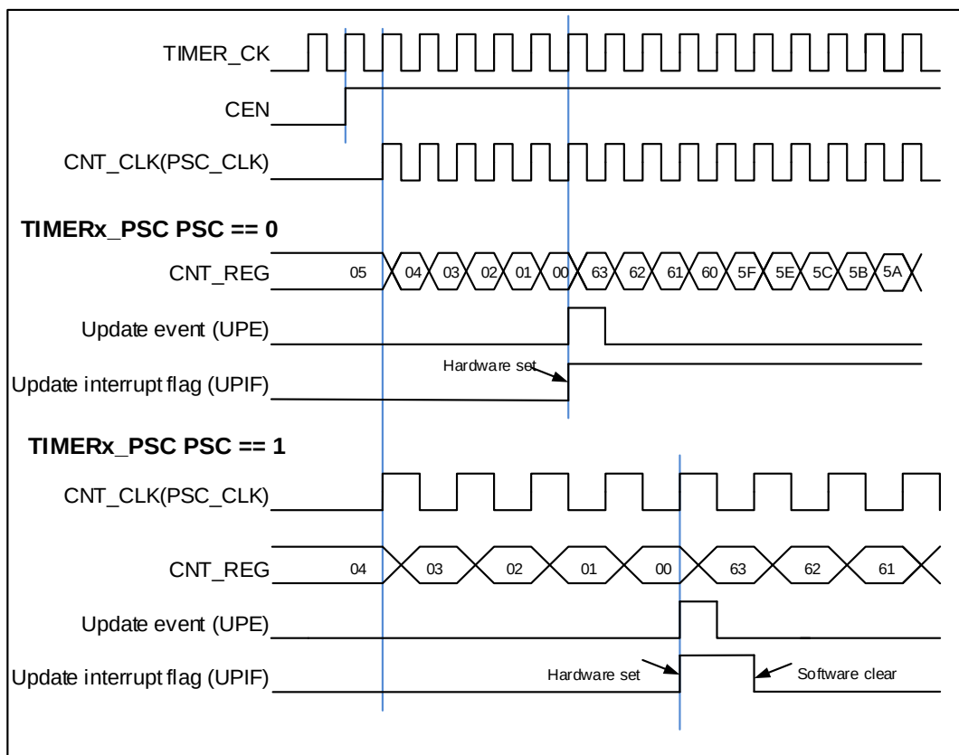
图 15-39. 向下计数时序图, PSC=0/1
