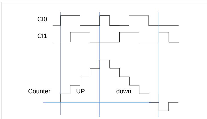
图 15-46. 编码器接口模式下计数器运行例子
