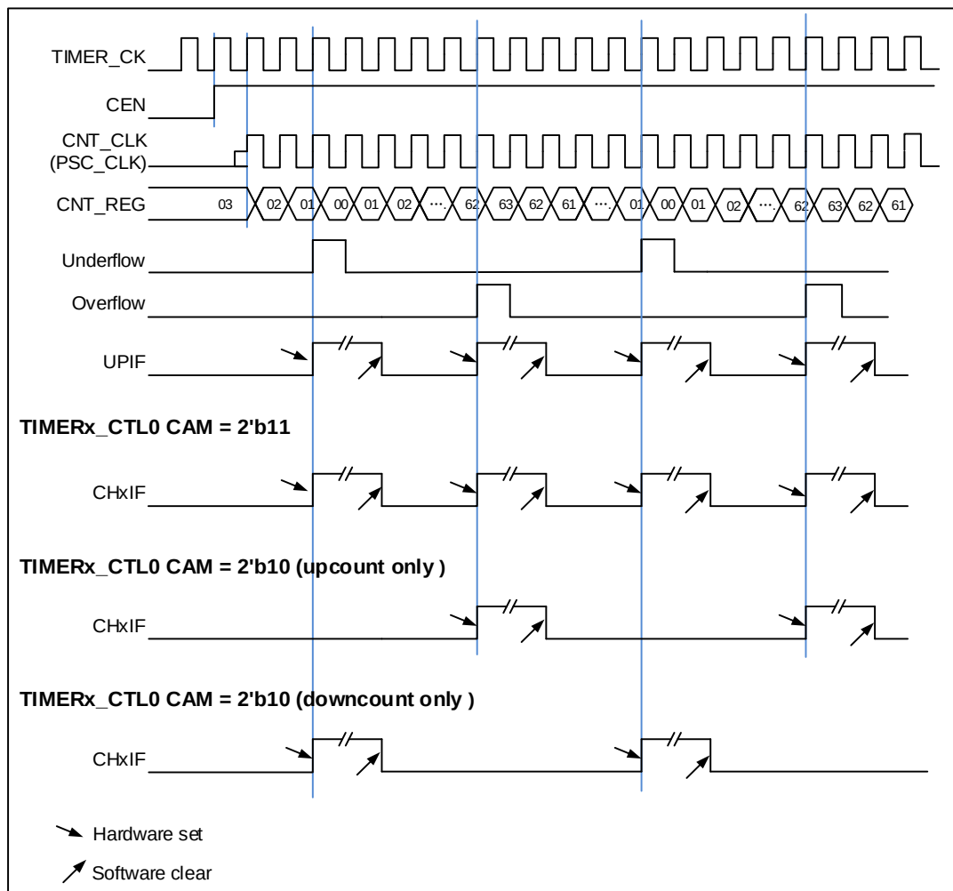
图 15-8. 中央计数模式计数器时序图
