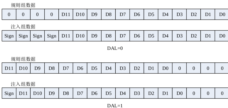
图 11-9. 12 位数据对齐
