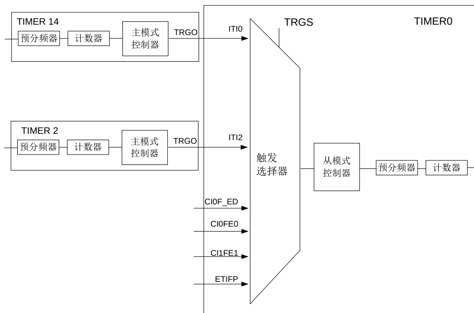
图 15-28. 定时器 0 主/从模式的例子
