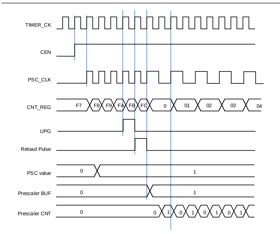
图 15-54. 当预分频器的参数从1变到2时,计数器的时序图
