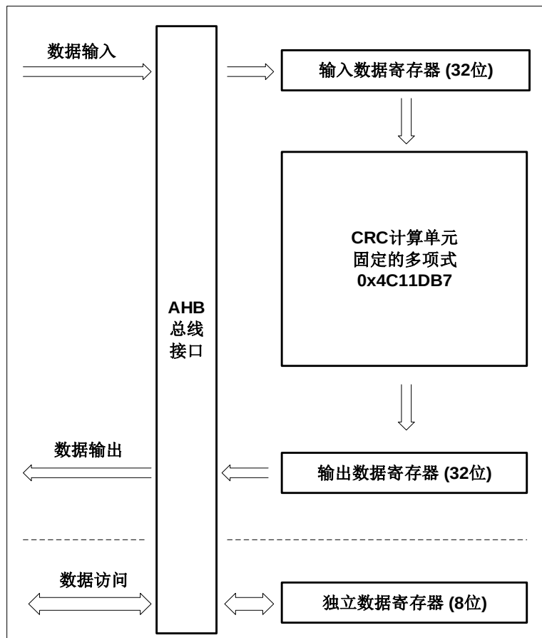
图 8-1. CRC 计算单元框图
