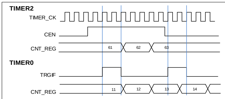
图 15-29. 用定时器 2 的使能信号触发定时器 0
