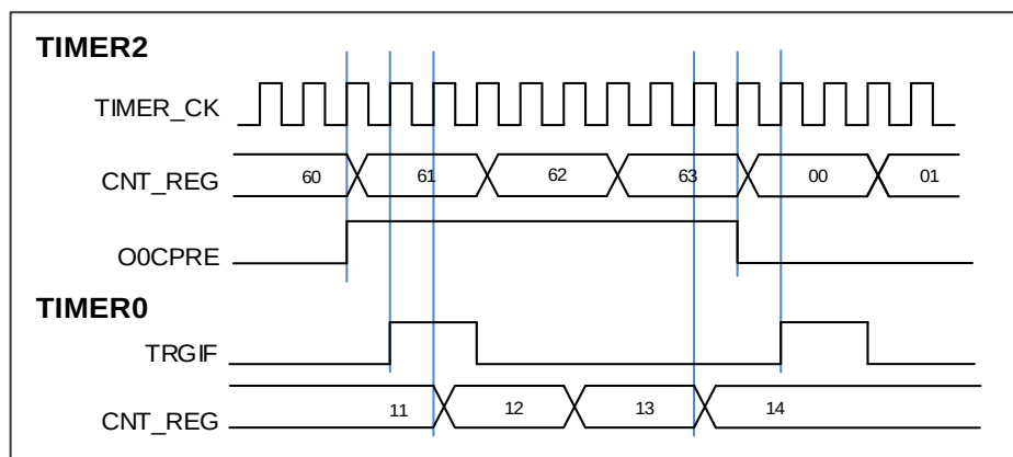
图 15-32. 用定时器 2 的 O0CPRE 信号控制定时器 0 的暂停模式
