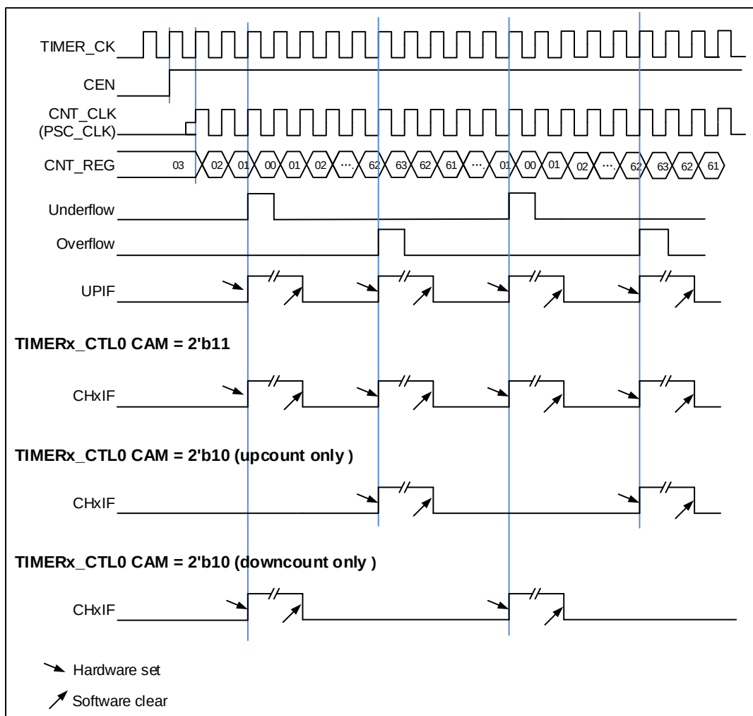
图 15-41. 中央计数模式计数器时序图
