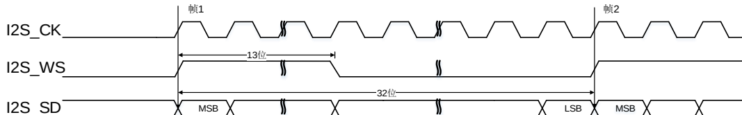
图 18-42. PCM 标准长帧同步模式时序图 (DTLEN=10, CHLEN=1, CKPL=0)
