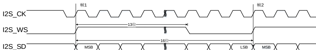
图 18-41. PCM 标准长帧同步模式时序图 (DTLEN=00, CHLEN=0, CKPL=1)
