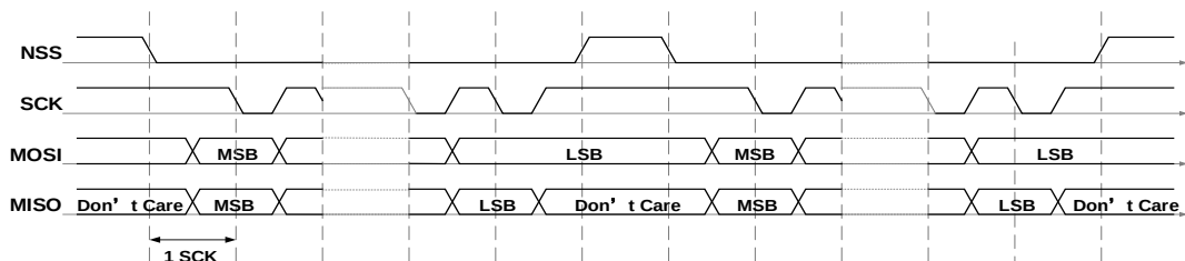
图 18-10. NSS 脉冲模式时序图（主机连续发送）
