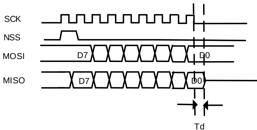
图 18-9. 从机 TI 模式时序图
