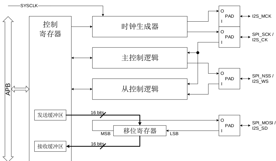
图 18-11. I2S 结构框图
