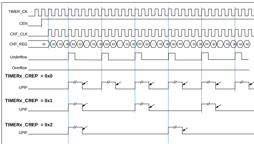
图 15-11. 在向下计数模式下计数器重复时序图
