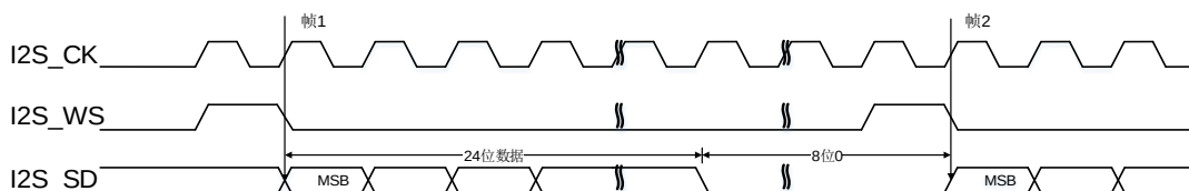
图 18-36. PCM 标准短帧同步模式时序图 (DTLEN=01, CHLEN=1, CKPL=0)
