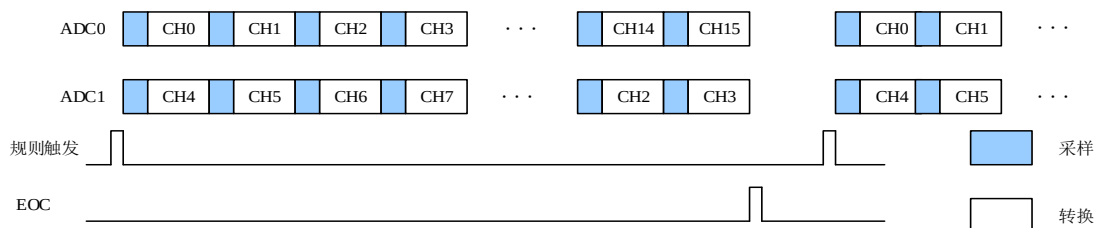
图 11-14. 基于 16 个通道的规则并行模式
