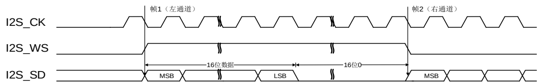
图 18-26. MSB 对齐标准时序图 (DTLEN=00, CHLEN=1, CKPL=0)
