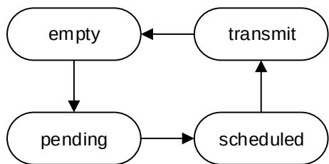
图 20-3. 发送邮箱状态转换
