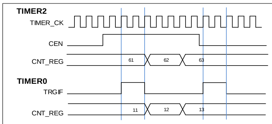
图 15-31. 用定时器2的使能信号来控制定时器0的暂停模式
