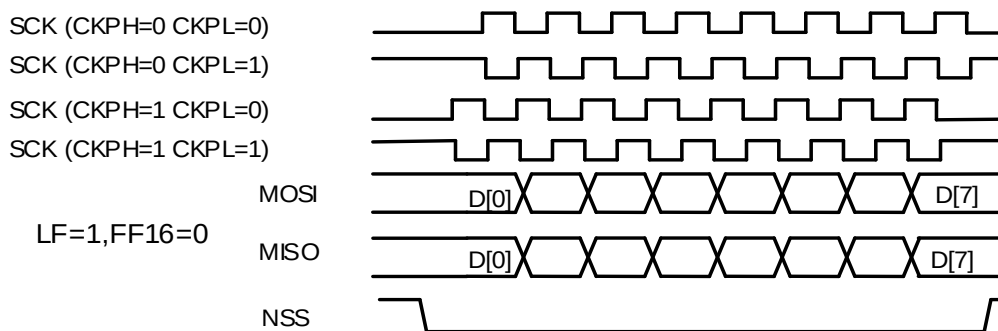
图 18-2. 常规模式下的 SPI 时序图
