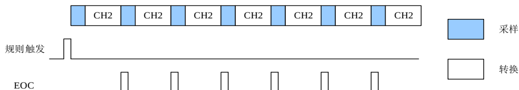
图 11-3. 连续转换模式
