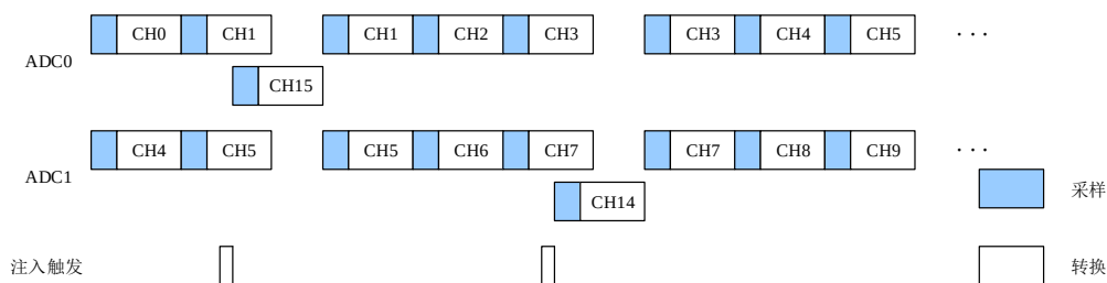
图 11-20. 规则并行和交替触发组合模式
