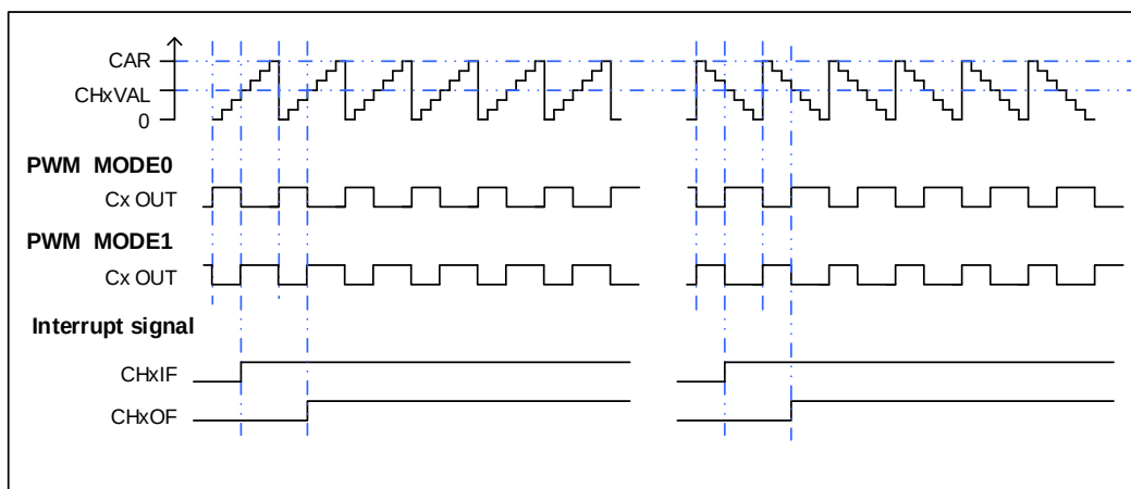
图 15-44. EAPWM 时序图
