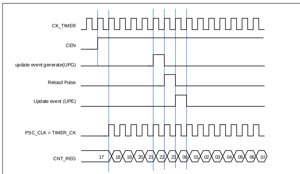
图 15-53. 内部时钟分频为1时正常模式下的控制电路
