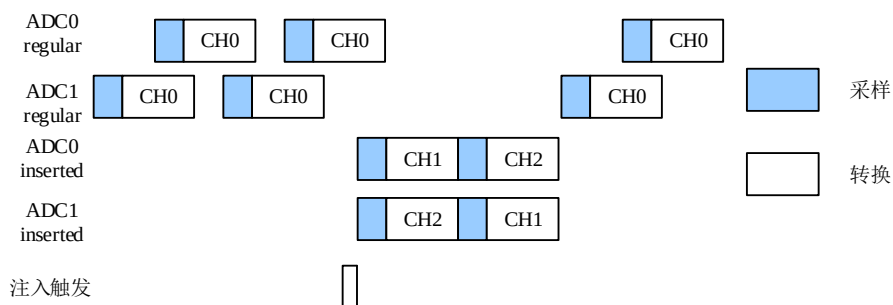
图 11-22. 交叉的单通道转换被注入序列 CH1 和 CH2 中断
