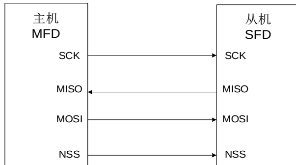
图 18-4. 典型的单工模式连接（主机：接收，从机：发送）
