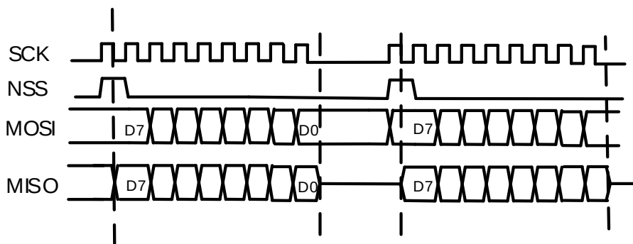
图 18-7. 主机 TI 模式在不连续发送时的时序图
