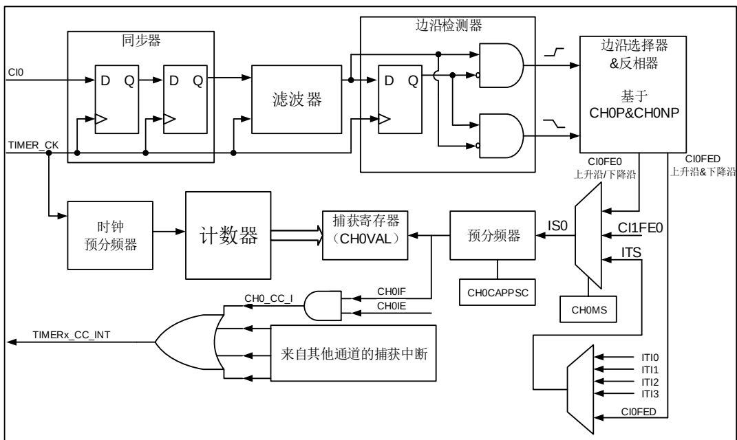
图 15-12. 输入捕获逻辑
