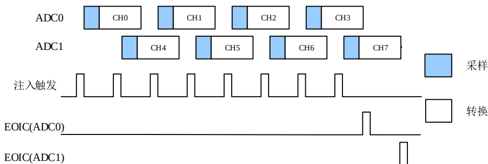
图 11-19. 交替触发: 间断模式下注入通道组
