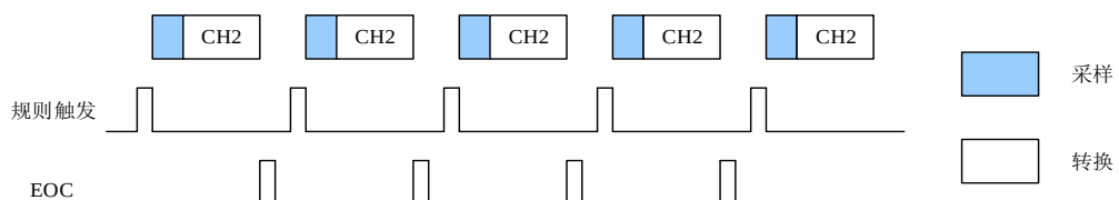
图 11-2. 单次转换模式
