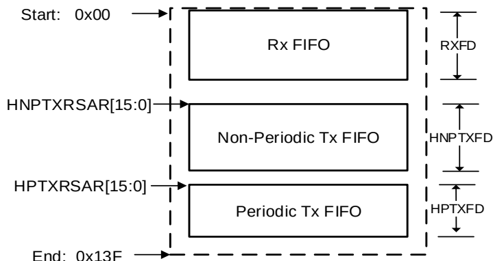
图 21-5. 主机模式 FIFO 空间
