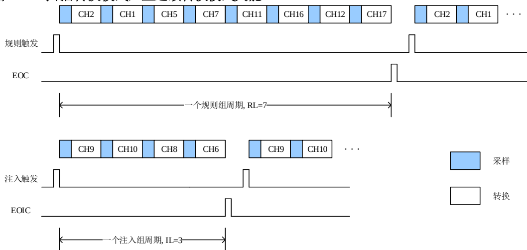
图 11-4. 扫描转换模式, 且连续转换模式失能
