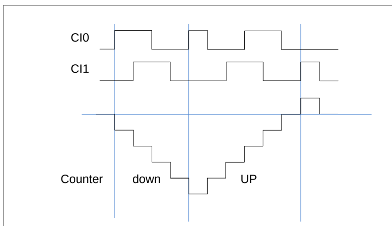
图 15-47. CI0FE0 极性反相的编码器接口模式下的例子
