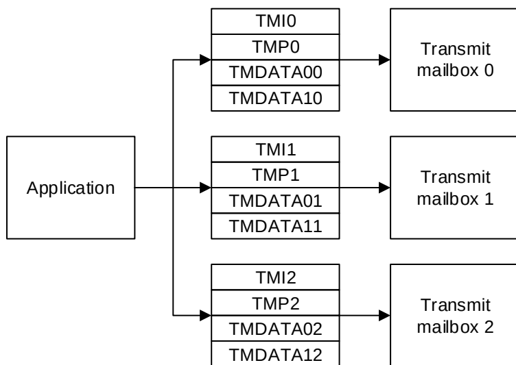
图 20-2. 发送寄存器
