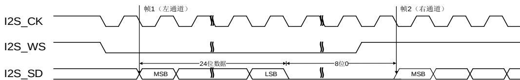
图 18-17. I2S 飞利浦标准时序图 (DTLEN=01, CHLEN=1, CKPL=1)
