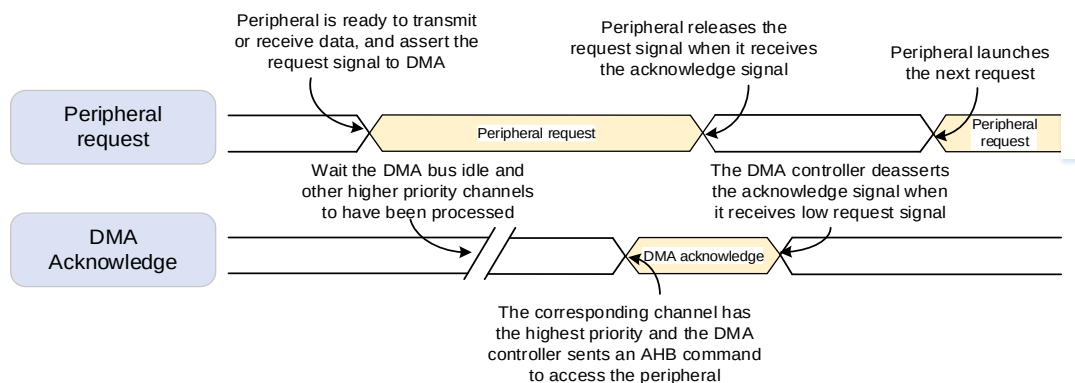
图 9-2. 握手机制
