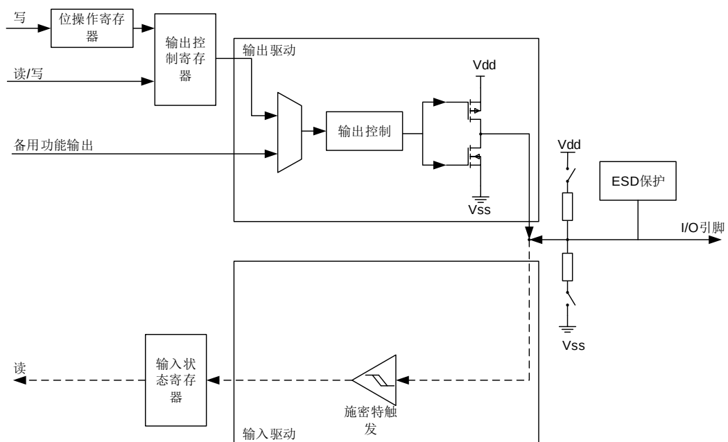
图 7-3. 输出配置
